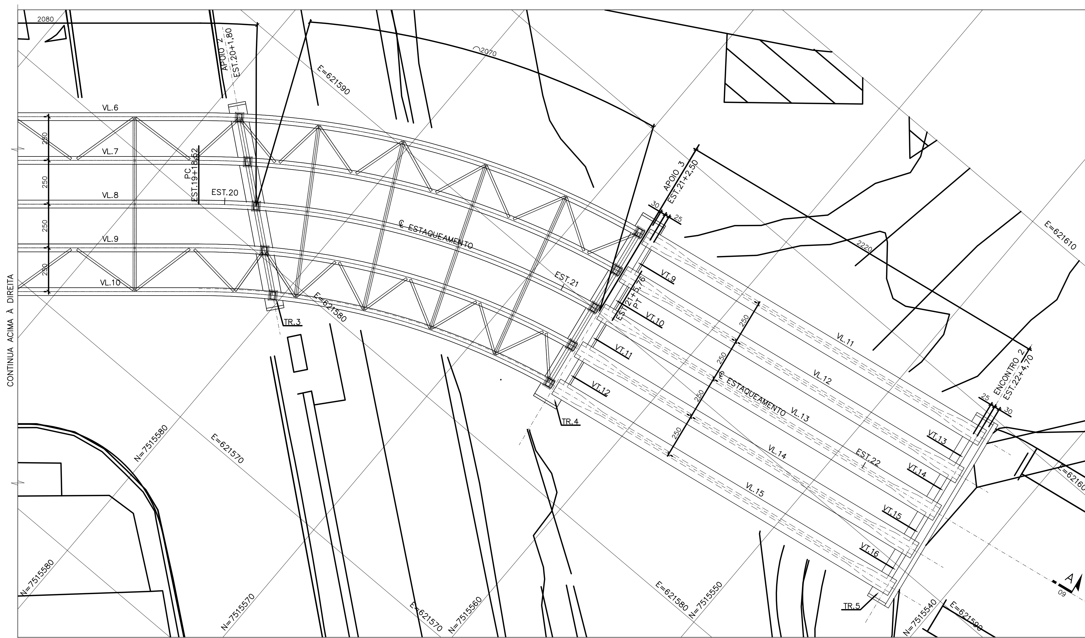
LOCAÇÃO DAS LONGARINAS E TRANSVERSINAS - PLANTA - (2ª PARTE) ESC 1:125
