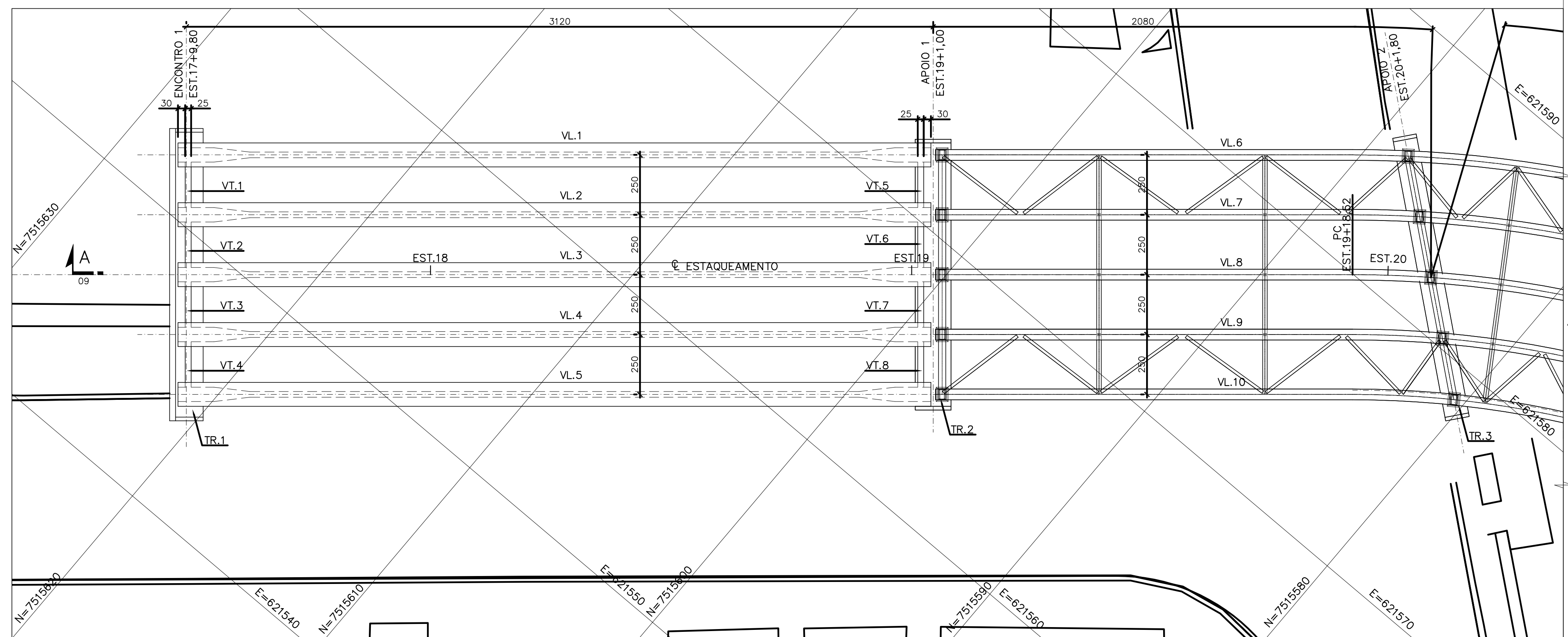
LOCAÇÃO DAS LONGARINAS E TRANSVERSINAS - PLANTA - (1ª PARTE) ESC 1:125
